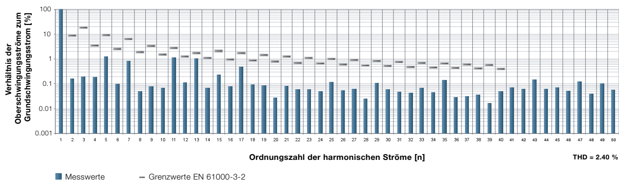
Oberschwingungsströme bei Nennleistung SolarMax 10MT2
