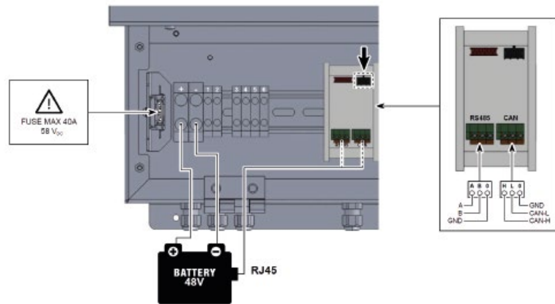
Typische RS485-Verkabelung
