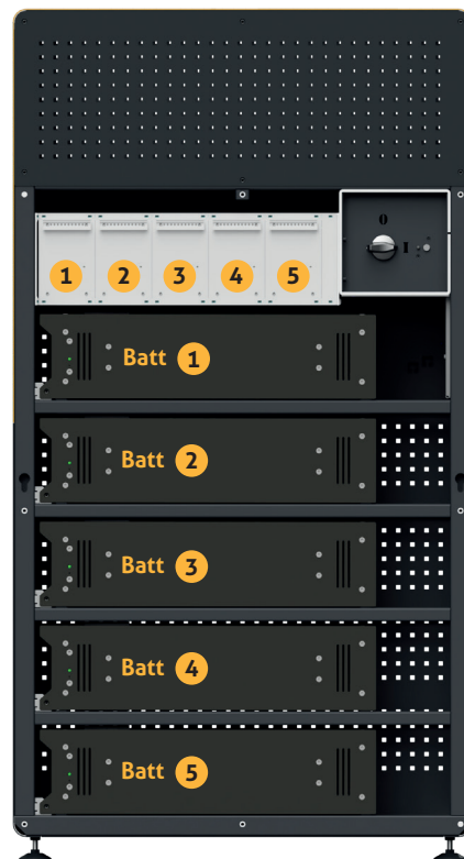
Abb. oben: MAX.STORAGE Ultimate 10 kW Lade/Entladeleistung 15 kWh Batteriespeicherkapazität
