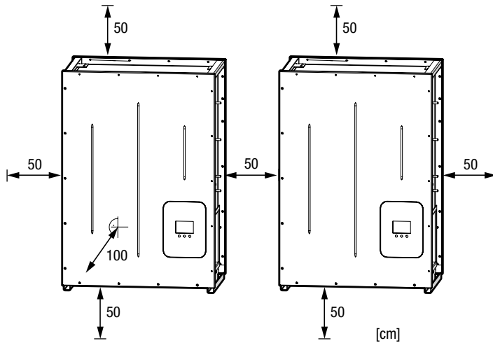
Bild 5 Minimale Montageabstände
