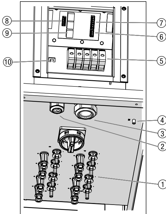
Bild 12 Anschlussbereich
