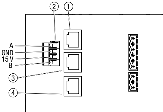
Bild 18 Netzwerkanschlüsse
