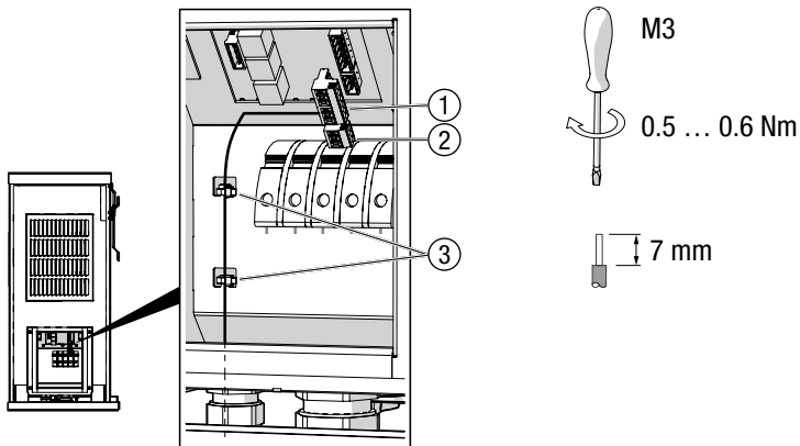
Bild 21 Statusmeldekontakte anschliessen
