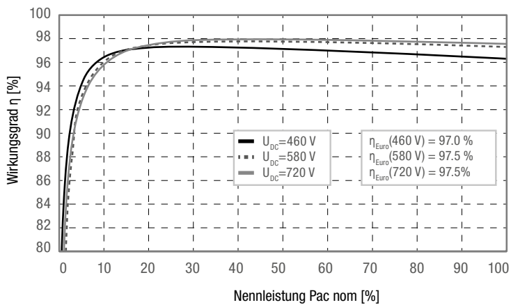
Bild 47 Wirkungsgradverlauf - SolarMax 30/32HT4
