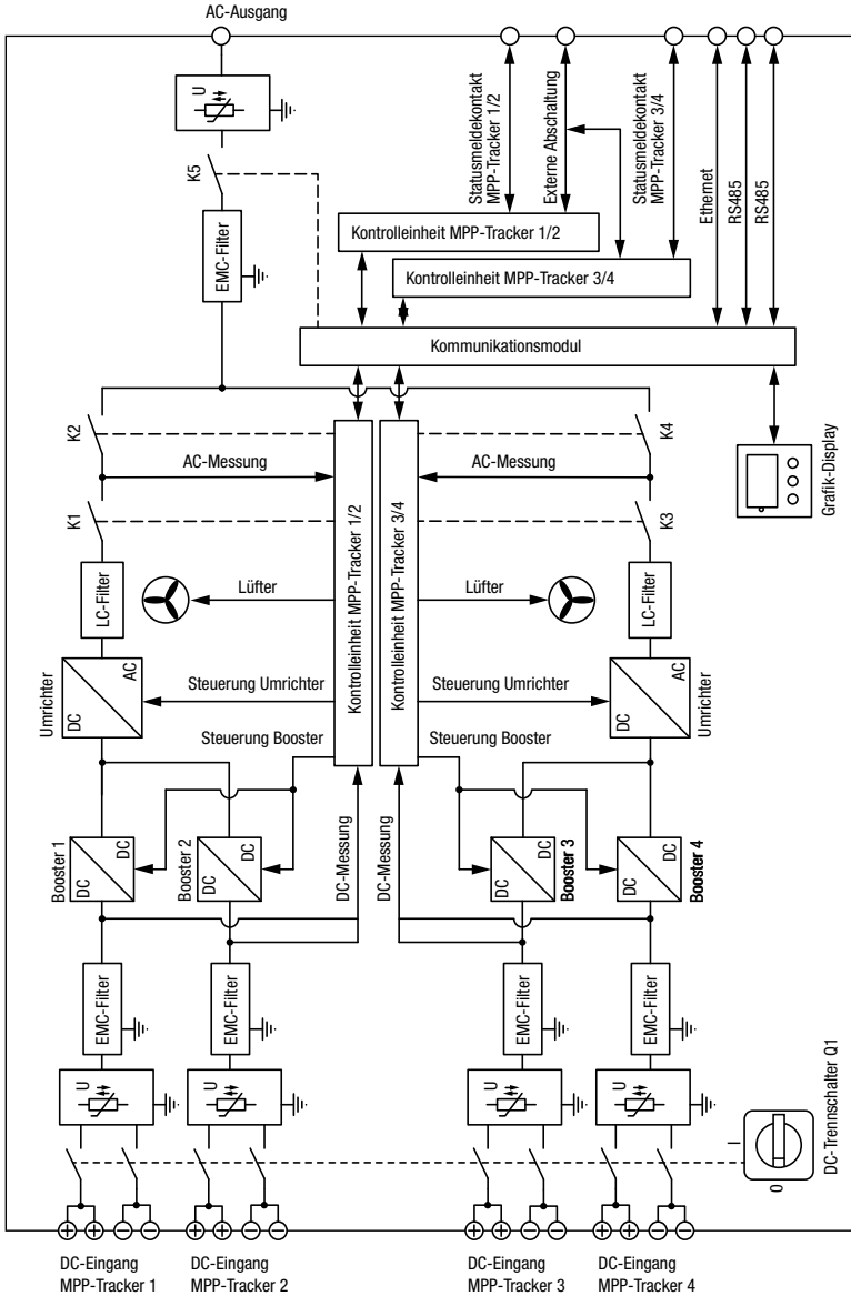
Bild 3 Blockschaltbild
