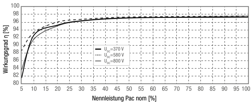
Bild 46 Wirkungsgradverlauf - SolarMax 25HT4
