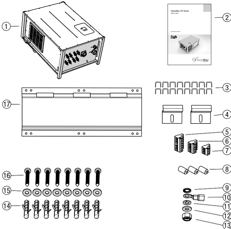
Bild 4 Lieferumfang
