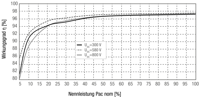
Bild 45 Wirkungsgradverlauf - SolarMax 20HT4
