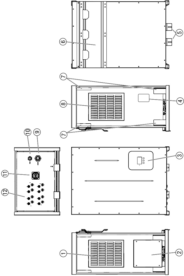
Bild 2 Außenansichten
