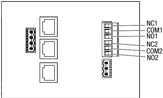
Bild 20 Statusmeldekontakte
