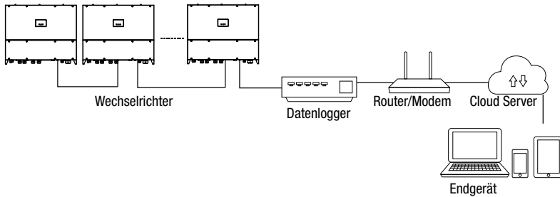
Abb. 18: RS485-Kommunikation mehrerer Wechselrichter
