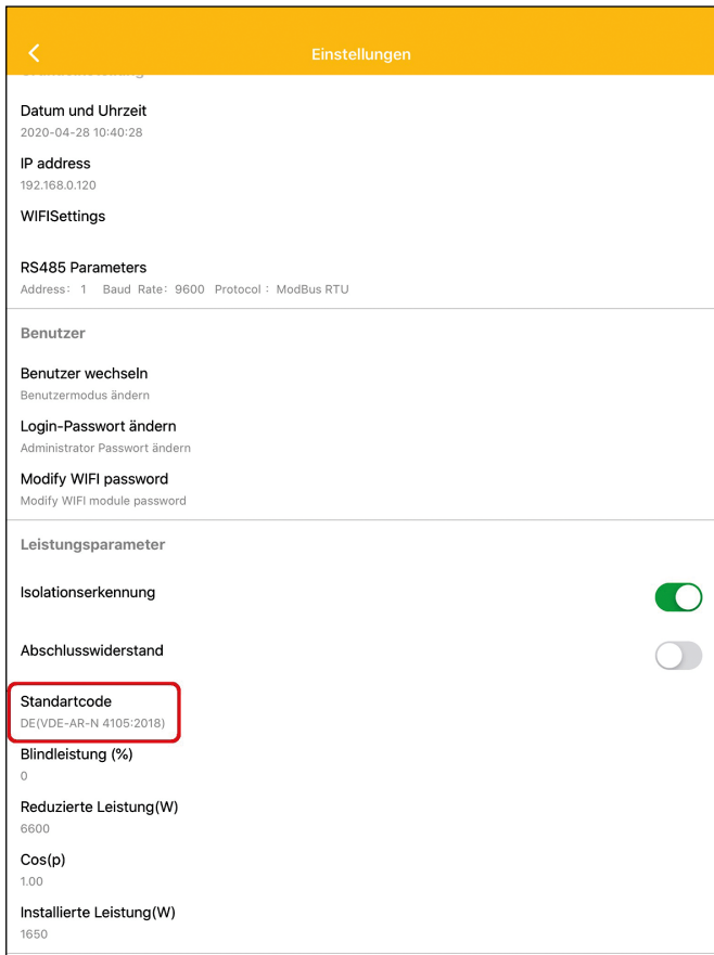
Abb. 24: MaxLink Wechselrichter-Einstellungen
