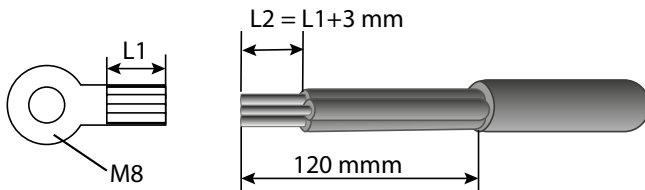
Abb. 14: Abisolieren des PV-Kabels
