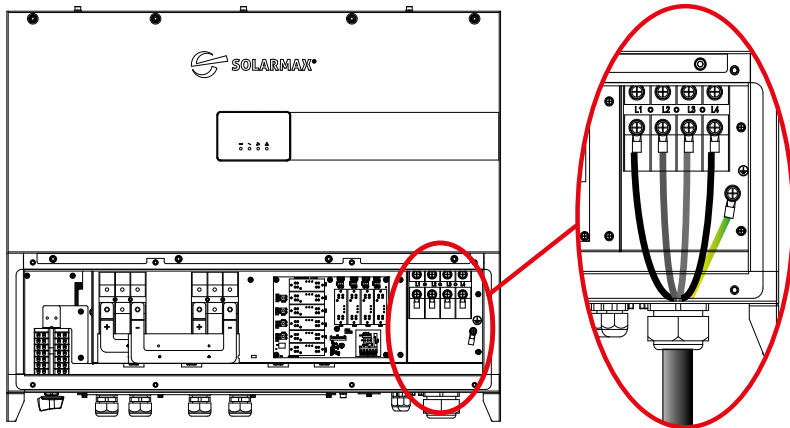
Abb. 13: Belegung der AC-Anschlussklemmen des Wechselrichters
