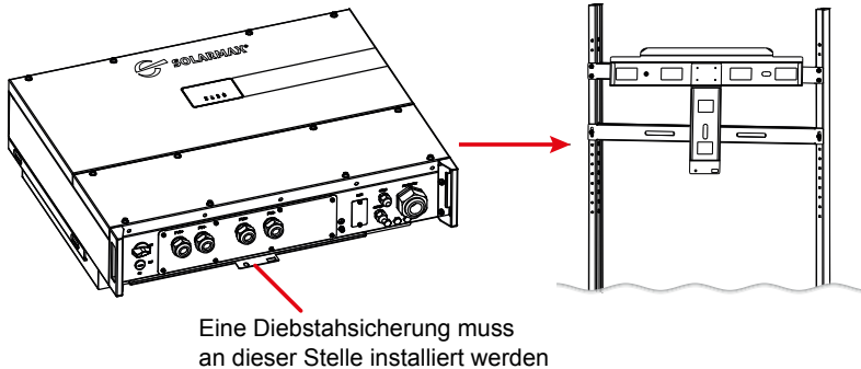
Abb. 8: Befestigen des Wechselrichter an einem Montagesystem
