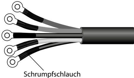
Abb. 12: Konfektionieren des AC-Kabels
