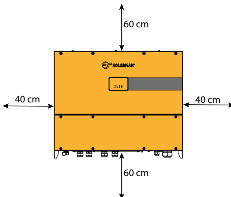
Abb. 5: Mindestabstände zum SHT-S-Gerät bei Montage
