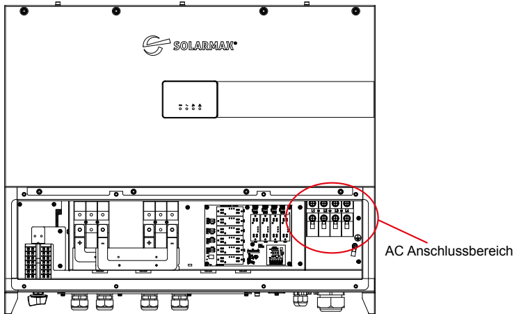
Abb. 11: Entfernen der Abdeckung des AC-Anschlusses
