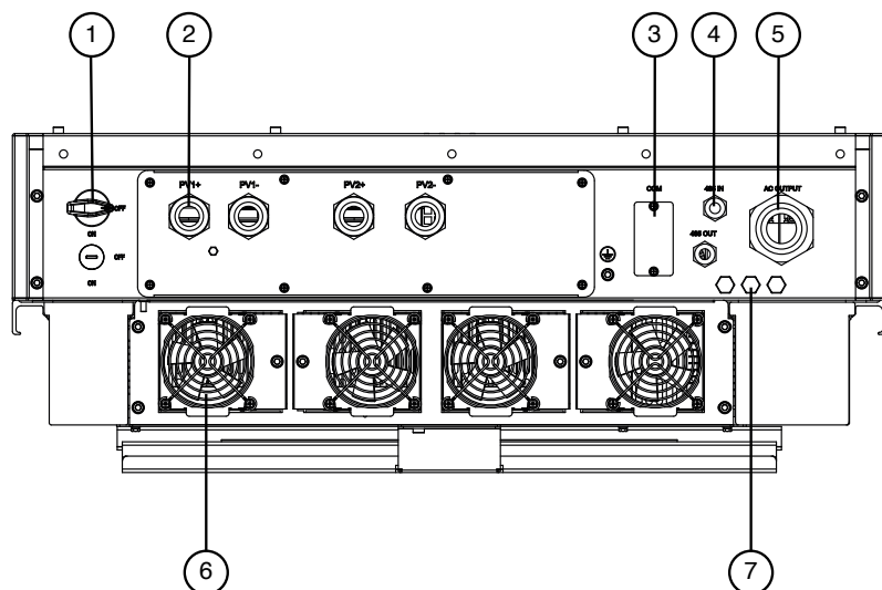
Abb. 3: Anschlüsse an der Unterseite des SHT-S-Gerätes
