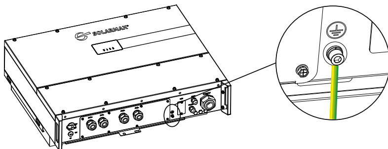
Abb. 10: Anschluss des externen Schutzleiters
