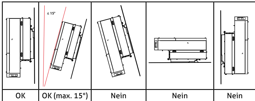
Abb. 6: Montageposition des SHT-S-Gerätes
