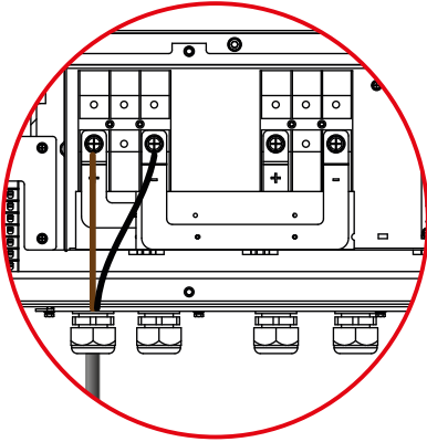
Abb. 17: Anschließen der PV-Kabel
