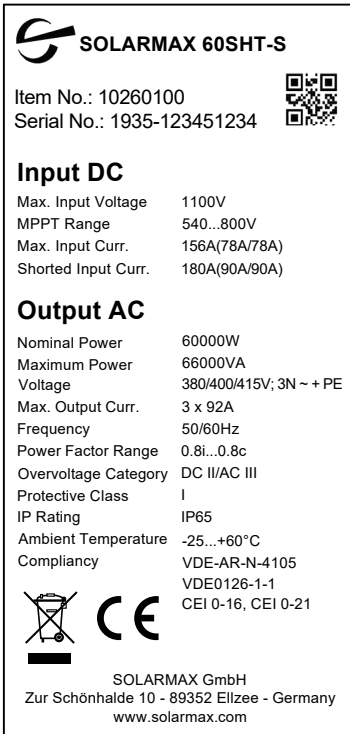
Abb. 1: Typenschild des SOLARMAX 60SHT-S
