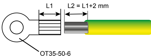
Abb. 9: Entfernen der Isolierung des Schutzleiters
