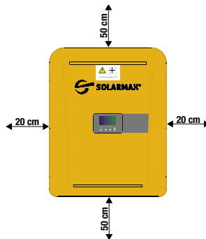
Abb. 6: Mindestabstände zum SMT-Gerät bei Montage
