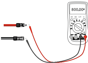
Abb. 21: Überprüfen der DC-Spannungswerte
