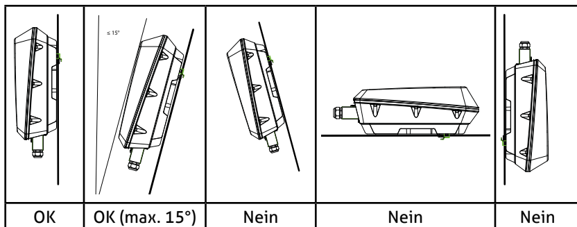
Abb. 7: Montageposition des SMT-Gerätes
