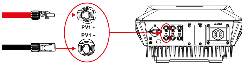
Abb. 22: Anschluss der konfektionierten Kabel an das SMT-Gerät
