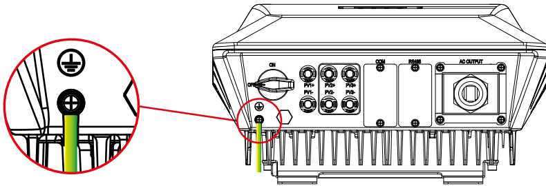
Abb. 15: Anschluss des externen Schutzleiters
