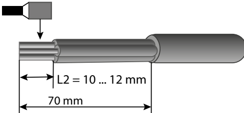
Abb. 10: Entfernen der Isolierung des AC-Kabels
