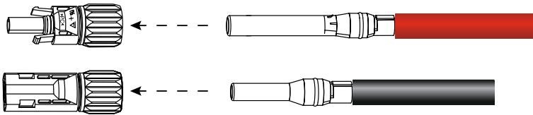
Abb. 19: Verbinden der Kontakte mit dem PVC-Gehäuse des Steckers
