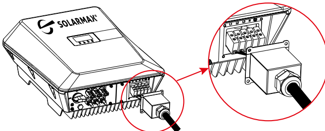
Abb. 12: Vorbereiten des AC-Kabels zum Anschluss an den Wechselrichter
