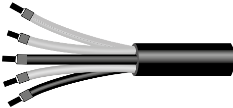
Abb. 11: Aderendhülsen des AC-Kabels
