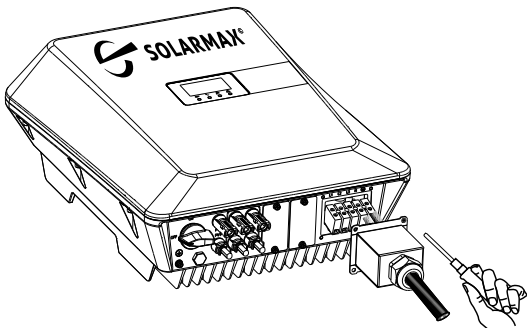
Abb. 14: Anbringen der AC-Kabelabdeckung
