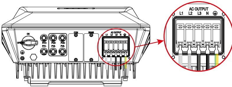
Abb. 13: Belegung der AC-Anschlussklemmen des Wechselrichters
