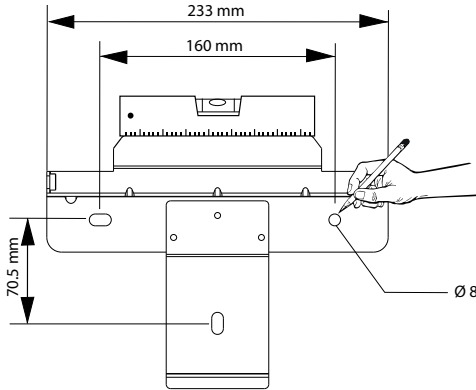
Abb. 8: Befestigen der Montageplatte an der Wand
