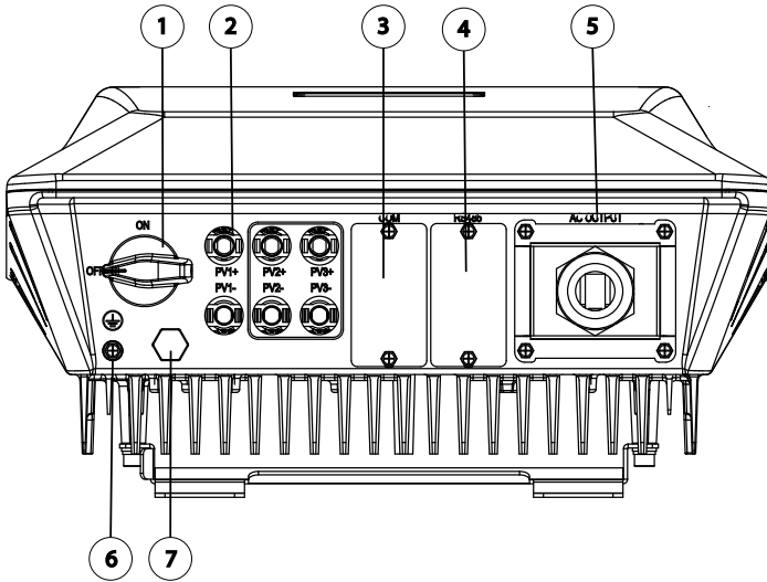
Abb. 4: Anschlüsse an der Unterseite des SMT-Gerätes
